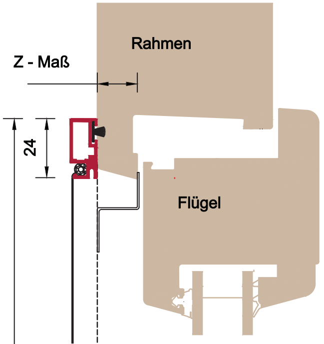
Vertikalschnitt SMB
