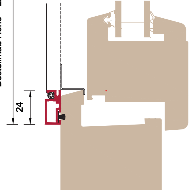
Vertikalschnitt SMB
