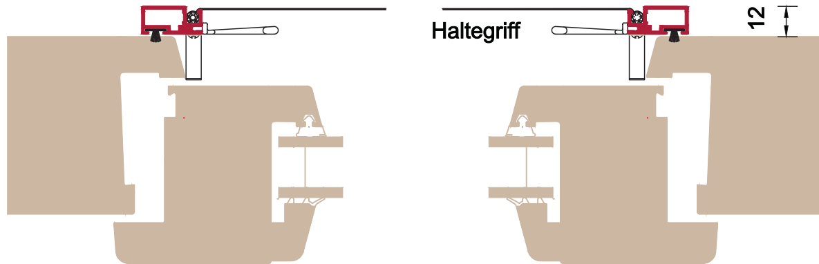
Horizontalschnitt SMB
